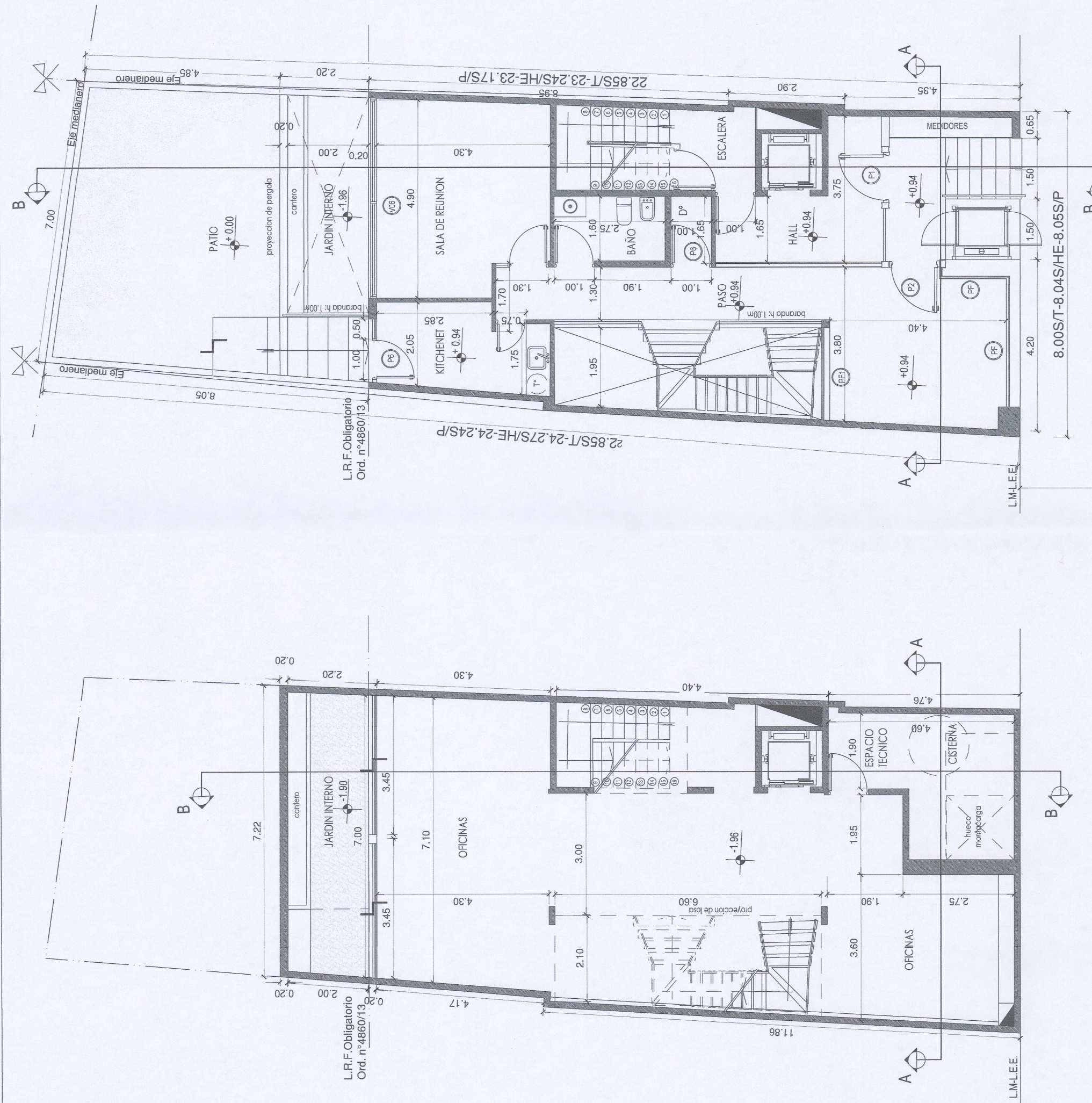
PLANTA SUBSUELO ESC: 1:100
