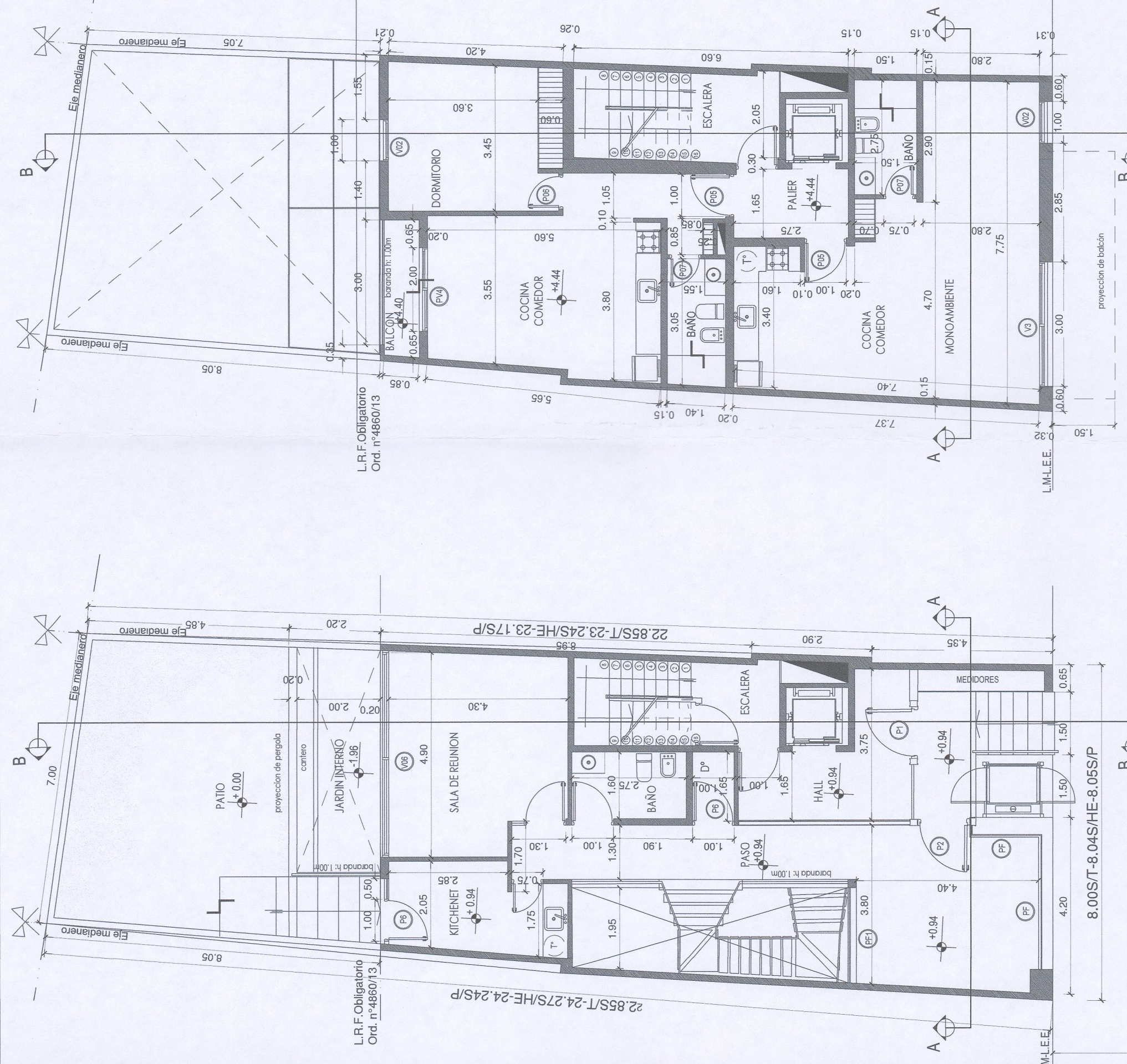
PLANTA 1° PISO ESC: 1:100
