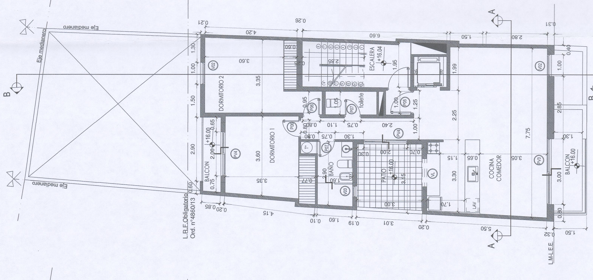
PLANTA 3° PISO ESC: 1:100
