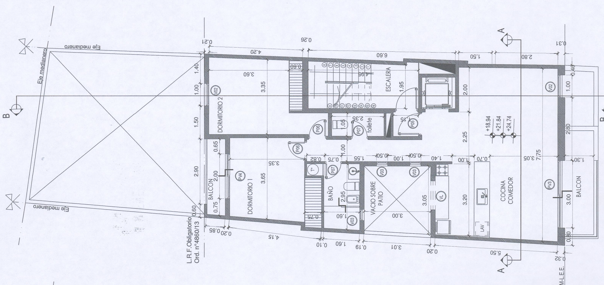
PLANTA 4° PISO ESC: 1:100
